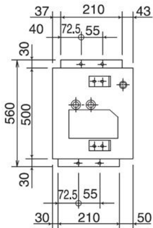
Чертежи внутреннего блока Panasonic S-F28DD2E5
