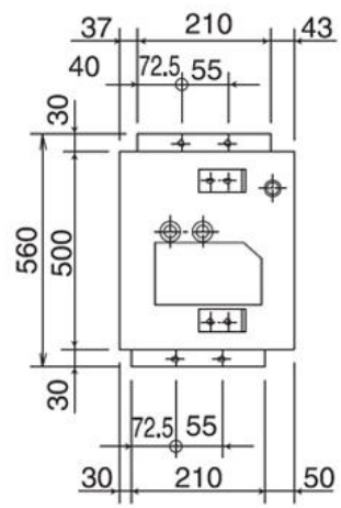
Чертежи внутреннего блока Panasonic S-F24DD2E5
