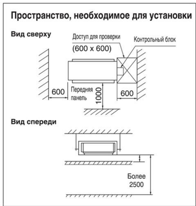
Чертежи внутреннего блока Panasonic S-F24DD2E5
